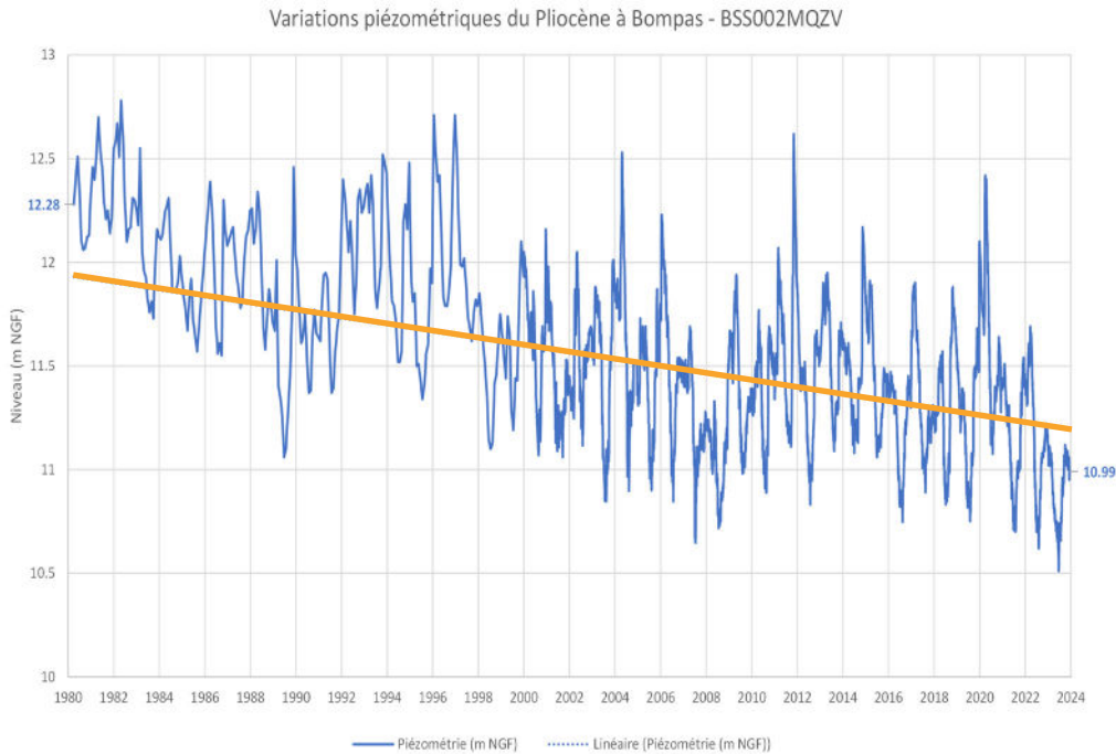
Relevés piézométriques de la nappe pliocène à Bompas. Le niveau de la nappe a baissé de 1,3 m depuis 1980.
